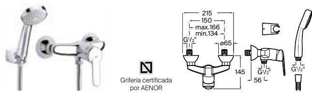
Grifería exterior para ducha Con ducha de mano Natura, flexible de 1,50 m y soporte fijo
