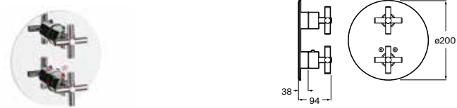
Grifería termostática empotrable para ducha Cromado A5A0743C00 € 749,00 Según tipo de instalación deberá colocarse una llave de paso
