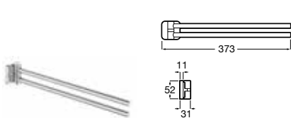
Toallero doble giratorio*
