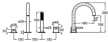
Grifería monomado de repisa para baño-ducha Con caño central, inversor, ducha de mano Stick y flexible de 1,60 m empotrable
