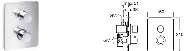
Grifería termostática empotrable para ducha A5A0679C00 € 660,00 Cromado
