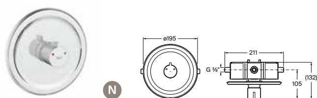
Grifería temporizada termostática empotrable para ducha Con rosetón Estándar A5A2579C00 € 437,00 Sist. Antilegionela A5A2G79C00 € 464,00 Cromado
