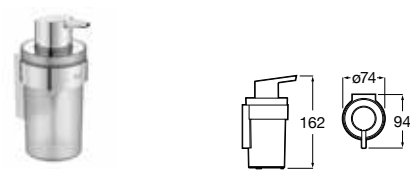
Dispensador jabón pared
