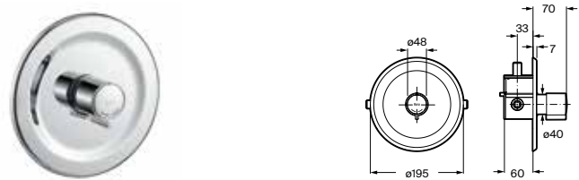
Grifería temporizada empotrable para ducha Con rosetón Estándar A5A2B79C00 € 392,00 Sist. Antilegionela A5A2H79C00 € 412,00 Cromado
