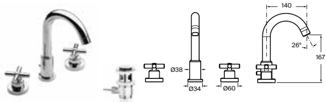
Grifería para lavabo Con caño central giratorio, aireador, desagüe automático y enlaces de alimentación flexibles Cromado A5A4443C00 € 508,00
