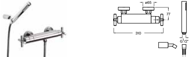
Grifería termostática exterior para ducha Con ducha de mano, flexible de 1,50 m y soporte articulado Cromado A5A1343C00 € 513,00
