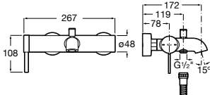
Grifería exterior para baño-ducha Con inversor automático
