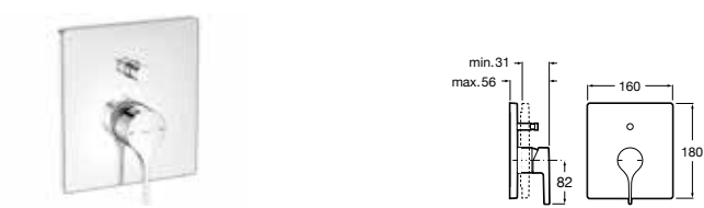
Grifería empotrable para baño- ducha A completar con: RocaBox ref. A525869403
