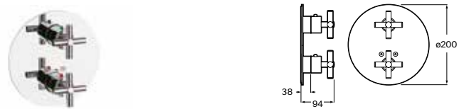
Grifería termostática empotrable para baño-ducha Con desviador-regulador de caudal Cromado A5A0643C00 € 773,00 Según tipo de instalación deberá colocarse una llave de paso
