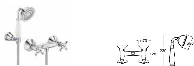
Grifería exterior para ducha Con ducha de mano, flexible de 1,50 m y soporte articulado Cromado A5A204BC00 € 241,00
