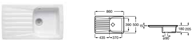
Beverly 85 E Fregadero reversible de una cubeta, un escurridor, dos orificios insinuados para la grifería y desagüe de 3½" Blanco 860 x 500 x 205 A366067000 € 340,00
