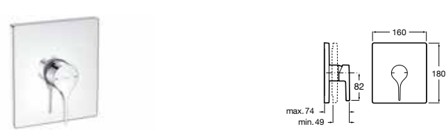
Grifería empotrable para baño o ducha A completar con: RocaBox ref. A525869403
